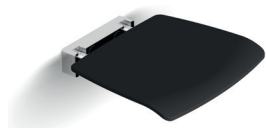
SN-0393 СКЛАДНАЯ МОДЕЛЬ СИДЕНЬЯ ДЛЯ КРЕПЛЕНИЯ НА СТЕНУ └ 371 x 377 x 65 мм Материал: алюминий ⚠ Нагрузка до 150 кг
