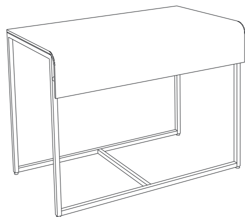
Art. 2040 Consolle senza lavabo Consola sin lavabo | Console without sink | Konsole ohne Waschbecken | Console sans lavabo cm 100 x 53 x h 73
