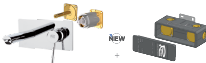
N 15 KB Miscelatore monocomando a incasso per lavabo, con piastra in ottone cromato da abbinare al box incasso.
