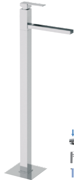
QC 18 Miscelatore monocomando lavabo da pavimento, con scarico click-clack con troppo pieno. Altezza 1010 mm, interasse 150 mm.
